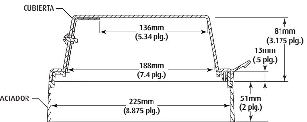
VISTA LATERAL MODELOS SIN SIRENA (Series STI-1200 y STI-3150)
